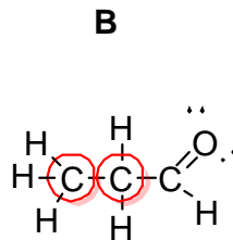
propanaali
