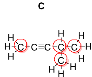
4-metyylipent-2-yyri
